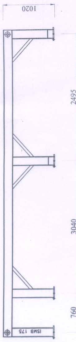
ELEVATION
